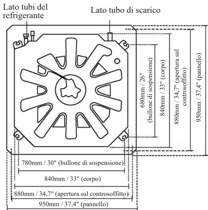
24-48K Modelli Classici dimensioni del foro sul controsoffitto
