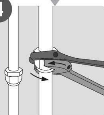
Conectar os canos do líquido refrigerante
